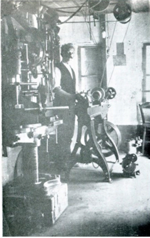
Halit Şazi , Erenköy'deki köşkünün arka bahçesinde kurduğu atölyesinde torna başında çalışırken, önde modelini, tornasını, tesviyesini kendi eliyle yaptığı motor görülmektedir (1916). 28
